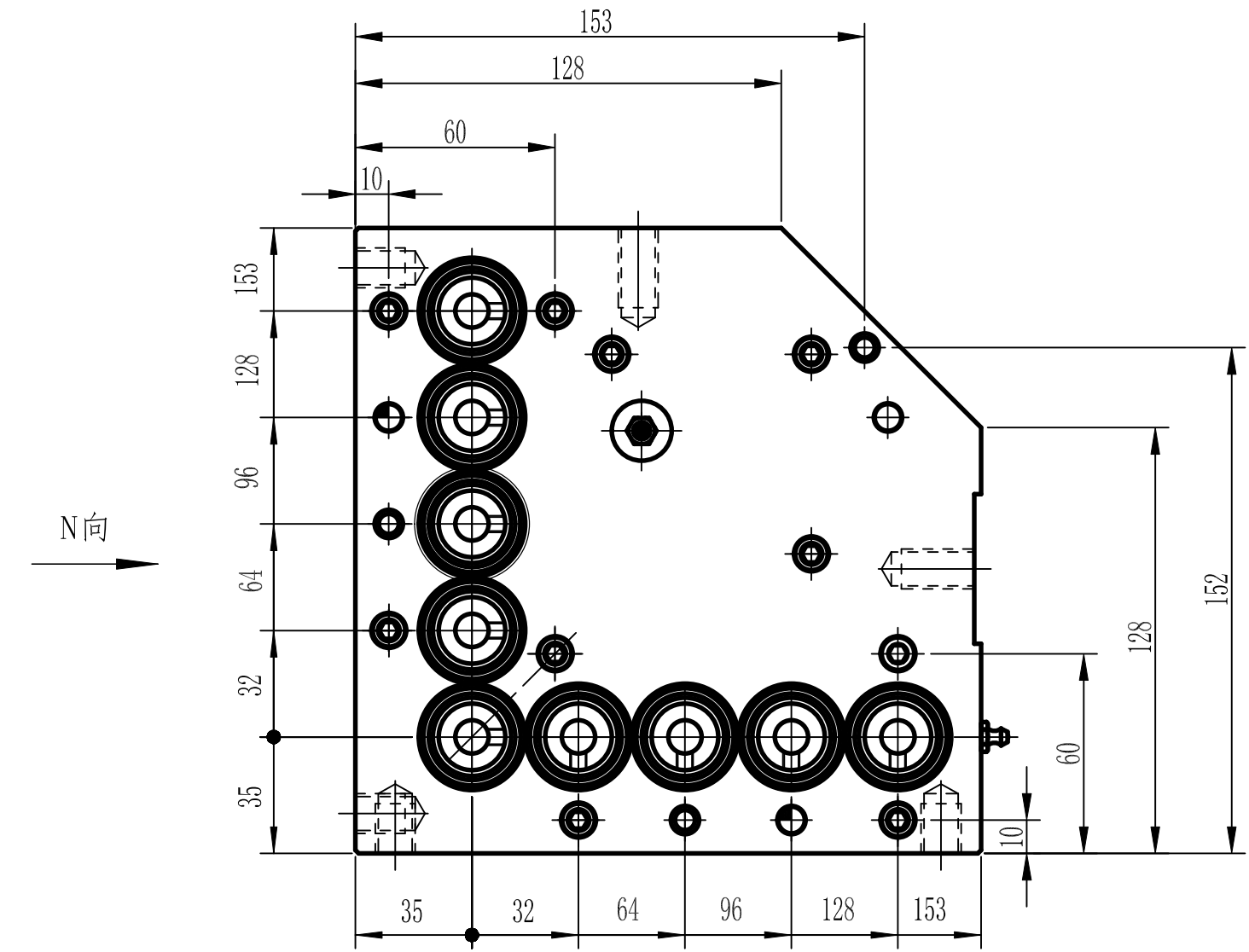
N向视图
