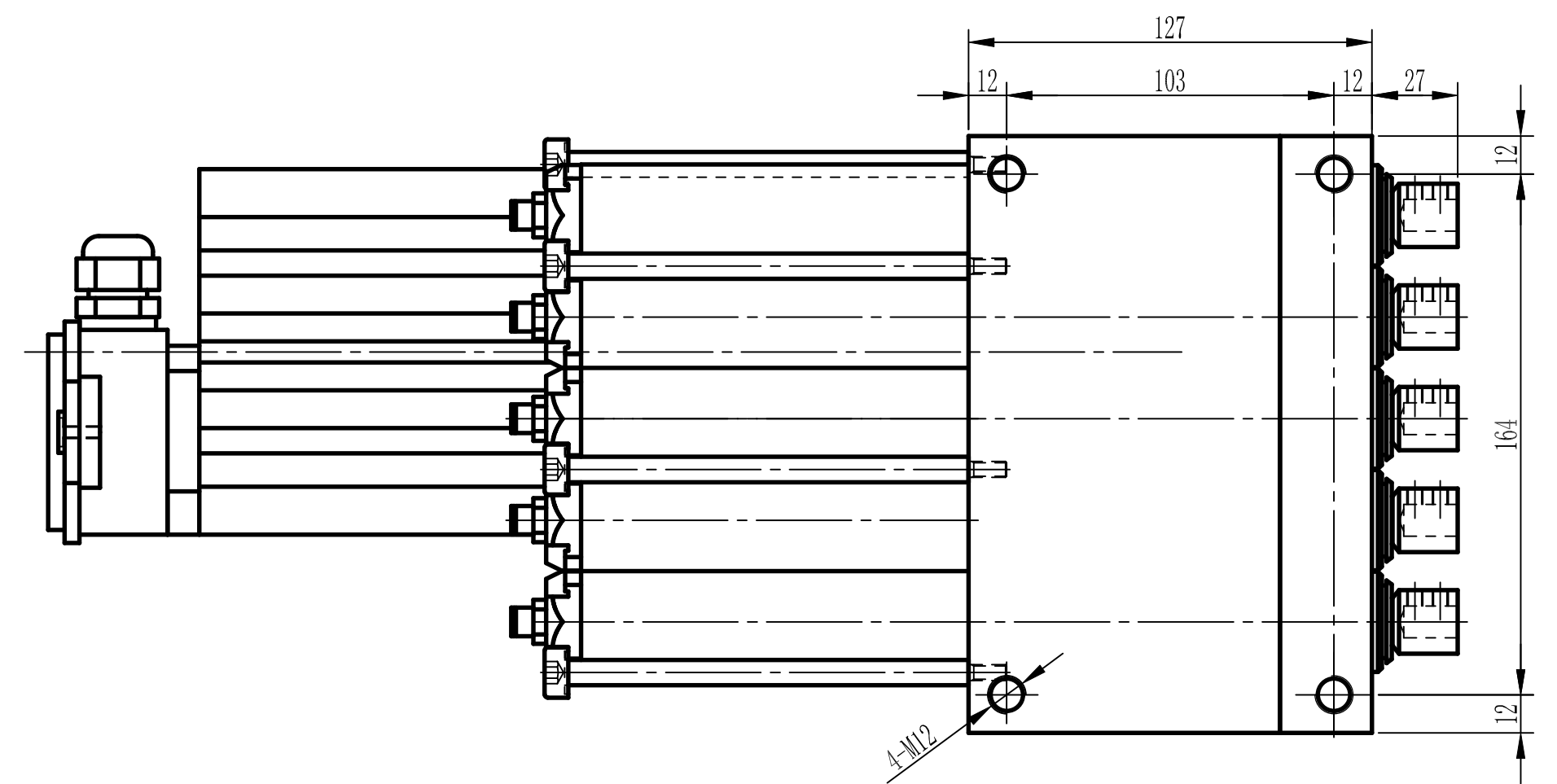
N向视图
